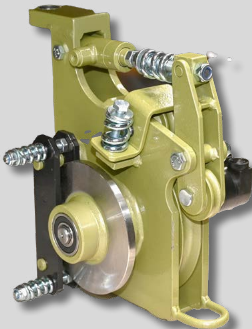
■ Hydraulischer Seilaustoß m. Seilverteiler
